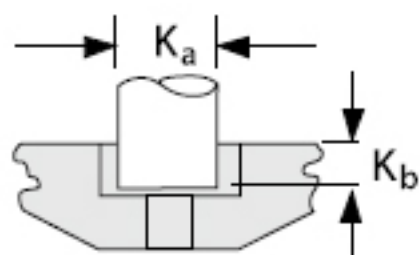
CD 外圈的定位销
