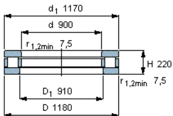
完整轴承
