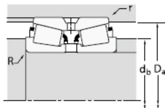
图3： DC外圈带一个润滑孔，设计为沉头孔形式，便于安装定位销。
