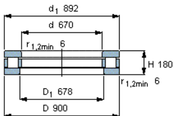
完整轴承
